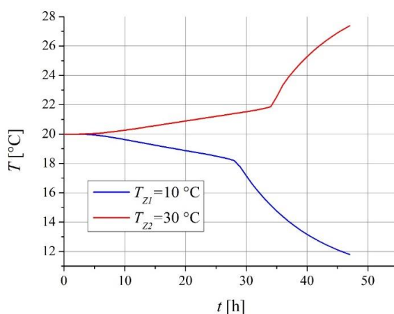
Slika 4: Temperatura ( T ) na notranji strani zidu A v odvisnosti od časa ( t ) pri konstantni zunanji temperaturi T_{Z2} = 30 °C (rdeča krivulja) in konstantni zunanji temperaturi T_{Z1} = 10 °C (modra krivulja).
