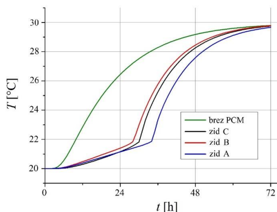
Slika 3: Temperatura ( T ) na notranji strani zidu v odvisnosti od časa ( t ) za zid brez PCM-ja (zelena krivulja), zid A (modra krivulja), zid B (rdeča krivulja) in zid C (črna krivulja) pri konstantni zunanji temperaturi T_{Z2} = 30 °C.
